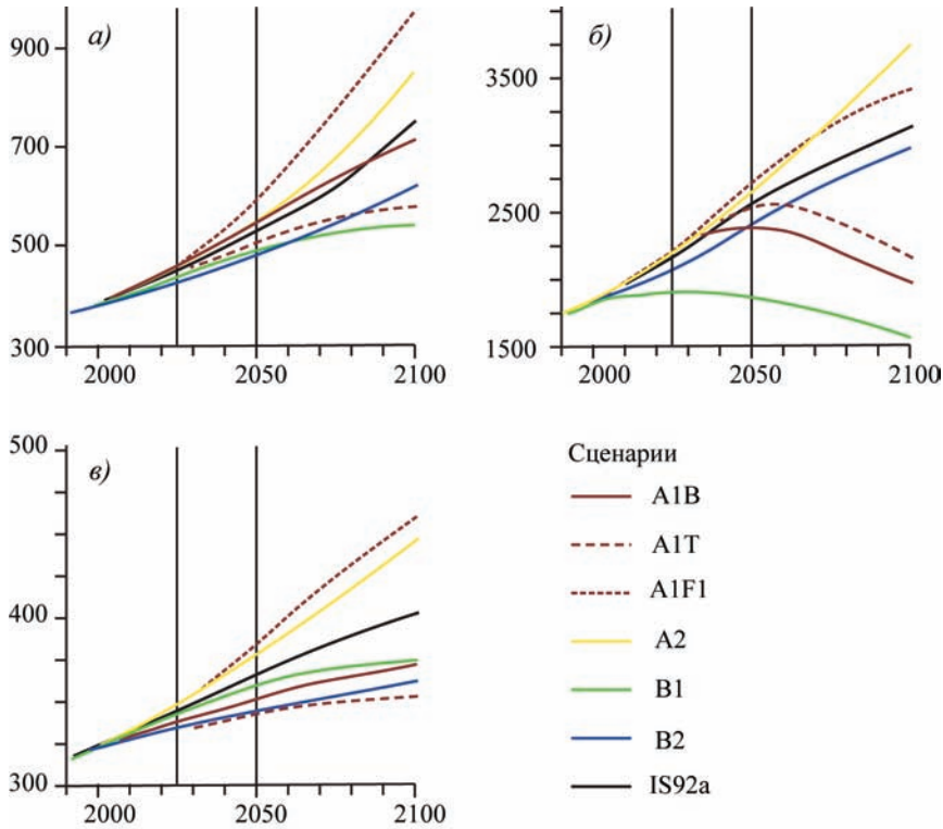
Рис. 8. Изменение среднегодовых среднеглобальных концентраций парниковых газов в приземном воздухе в XXI веке по указанным сценариям их антропогенных эмиссий.
